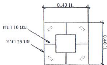
แบบขยาย Plate ปิด NOT TO SCALE
