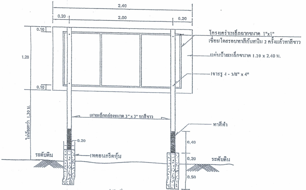
รูปตัดด้านหลัง scale nts.
