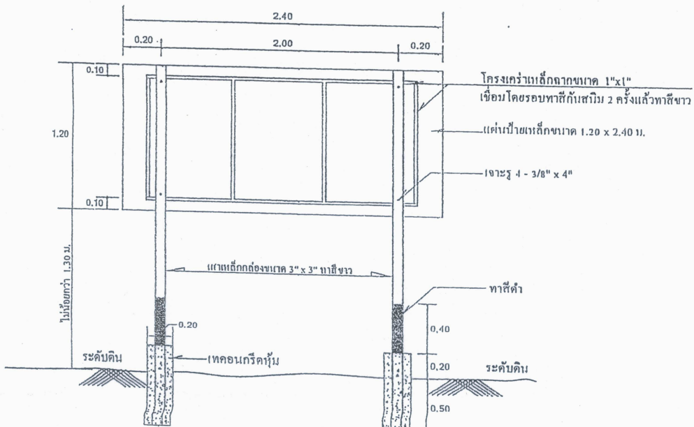
รูปตัดด้านหลัง scale 1/15
