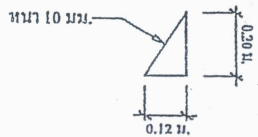
แบบขยายแผ่น Plate ชัด โคนเสา NOT TO SCALE
