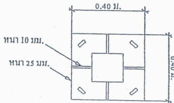
แบบขยาย Plate เสา NOT TO SCALE
