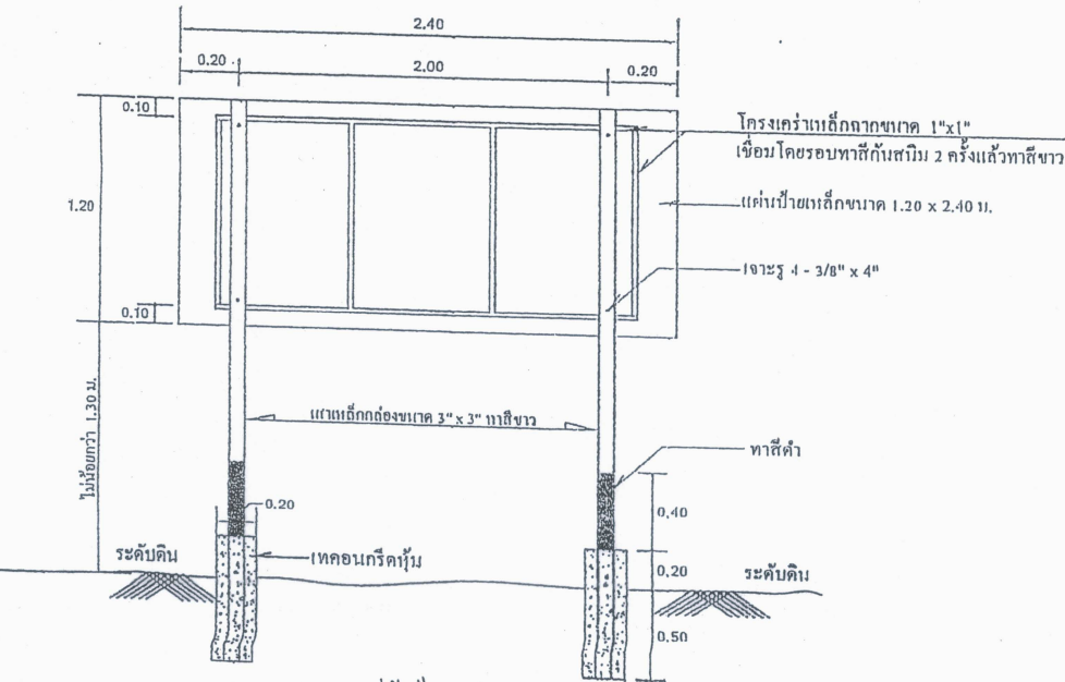
รูปตัดด้านข้าง scale 1/15
