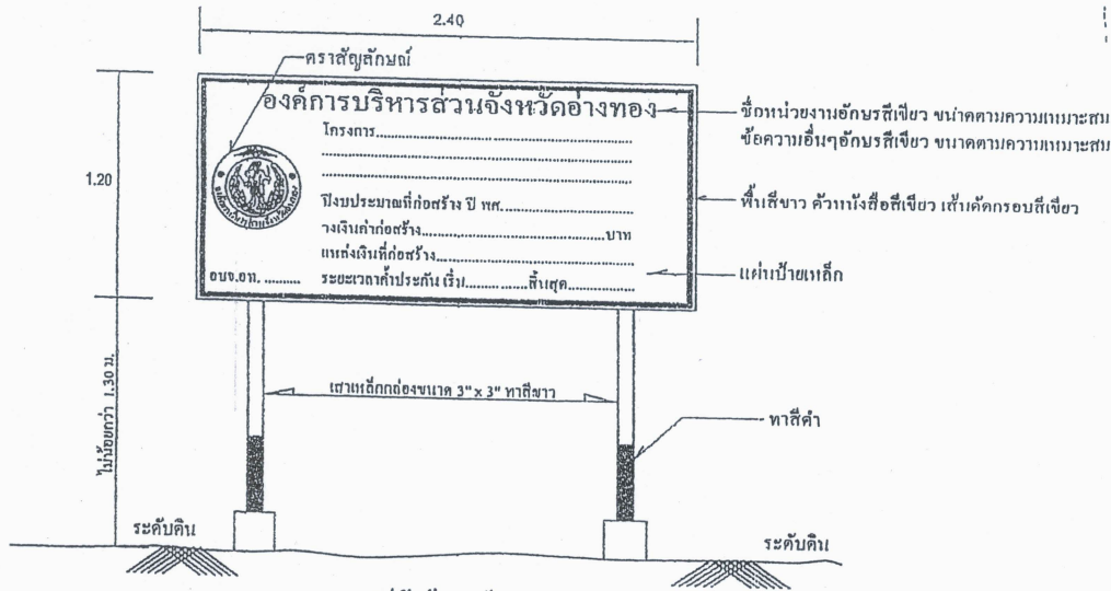
รูปตัดด้านหน้า scale 1/15
