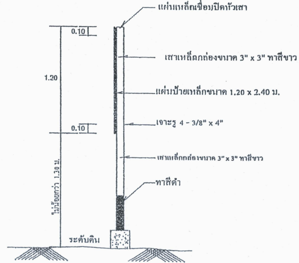
รูปตัดด้านข้าง scale 1/15
