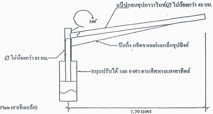
แบบขยายท่อน้ำ NOT TO SCALE
